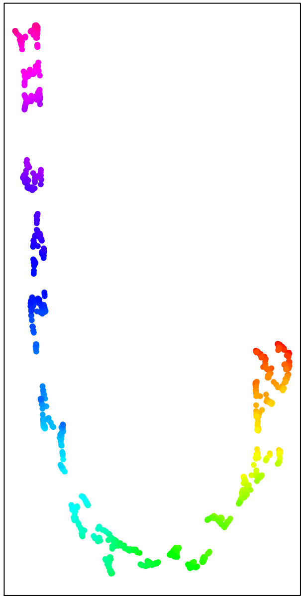
UMAP (uwot)
