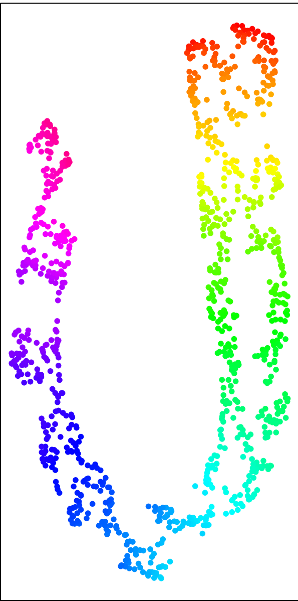
t-SNE (tapkee)
