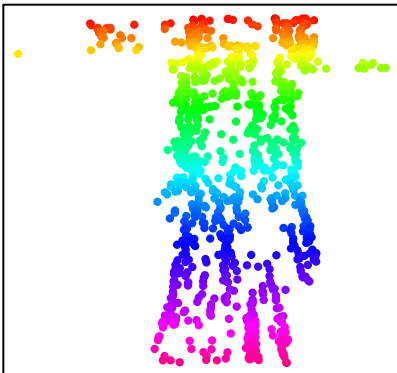
Isomap
