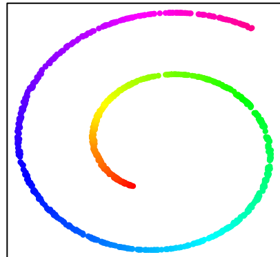
PCA
