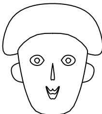
fluviatile
